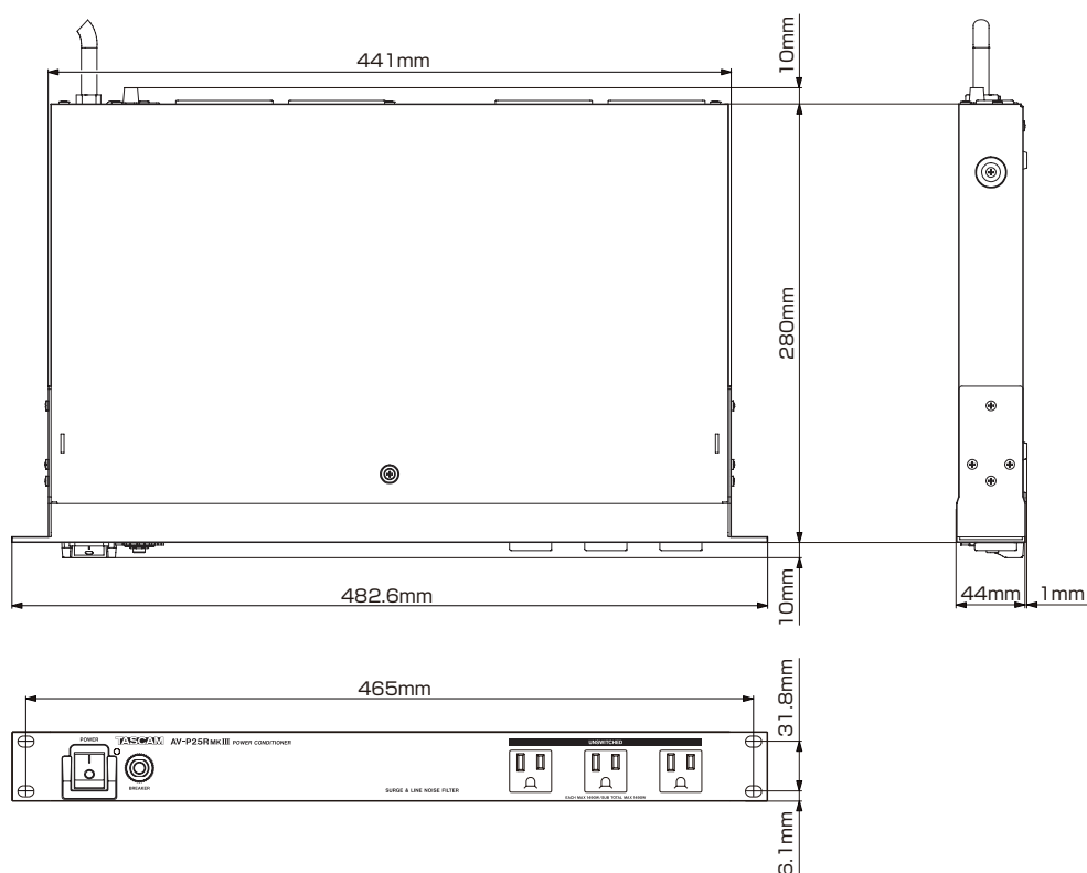
[例：AV-P25RMKIIIの寸法図]
