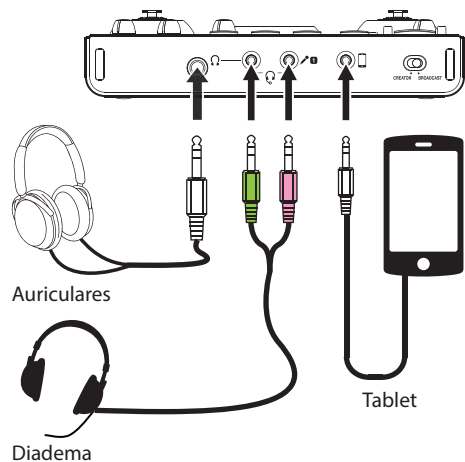
Ejemplos de conexión de un MiNiSTUDIO (panel frontal)
