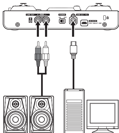
Monitores autoamplificados con conectores RCA
