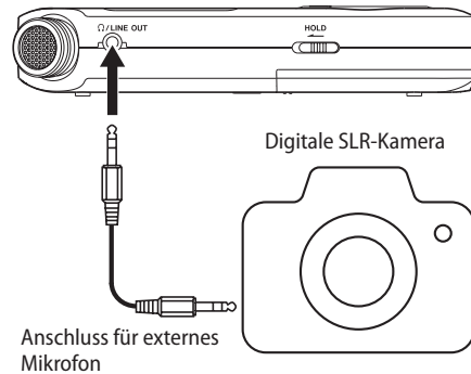
Anschlussbeispiel
