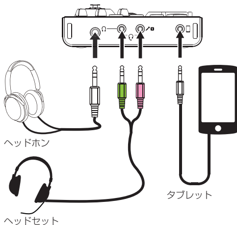
[MiNiSTUDIOを使った接続例 (フロントパネル)]
