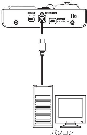
[MiniSTUDIOを使った接続例（リアパネル）]
