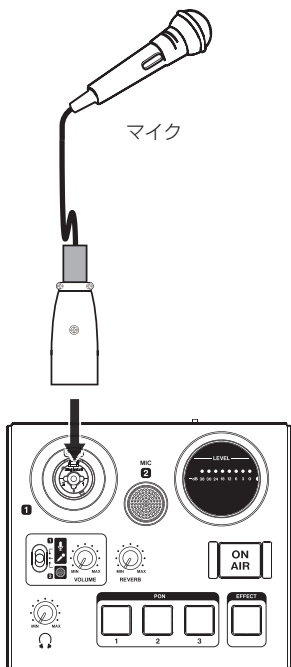
[MiNiSTUDIOを使った接続例 (トップパネル)]
