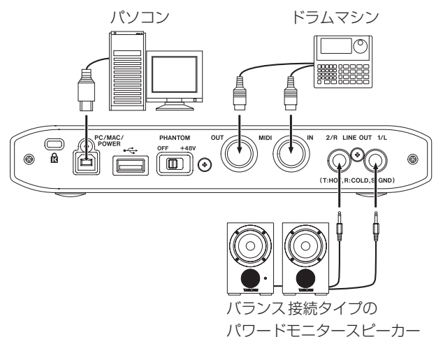
[ パソコン使用時の接続例 (リアパネル) ]
